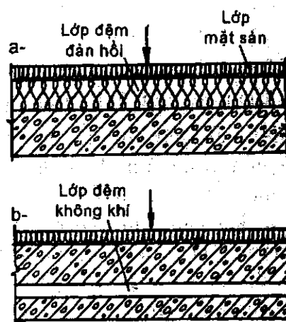
Hình 8.37 : Các sơ đồ kết cấu sàn giữa các tầng
