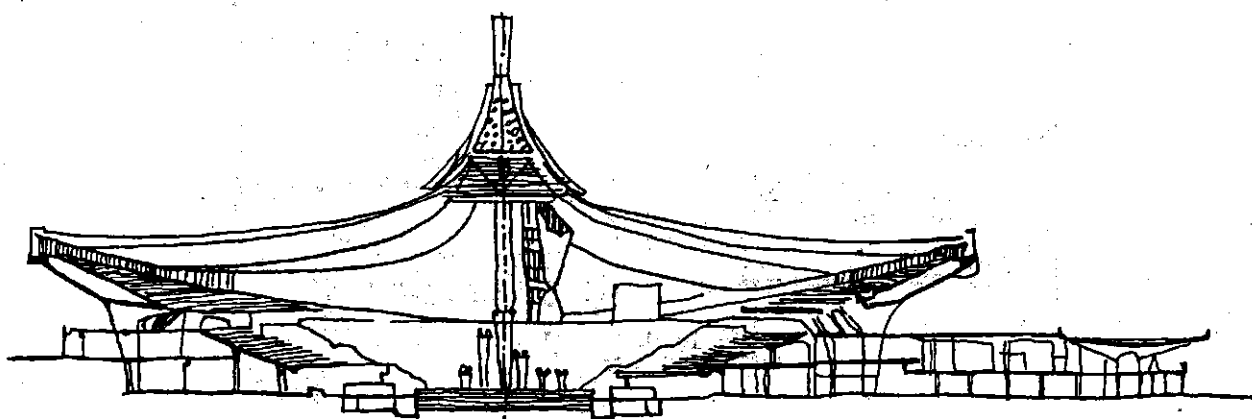
MẶT CẮT NHÀ THI ĐẤU
