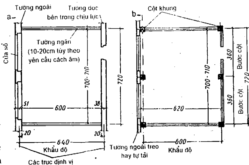
Hình 5.8 : Gắn kích thước của phòng với hệ kết cấu của nhà
