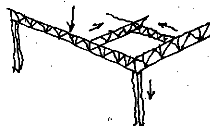
Hình 6.3 : Hệ khung - cột giàn
