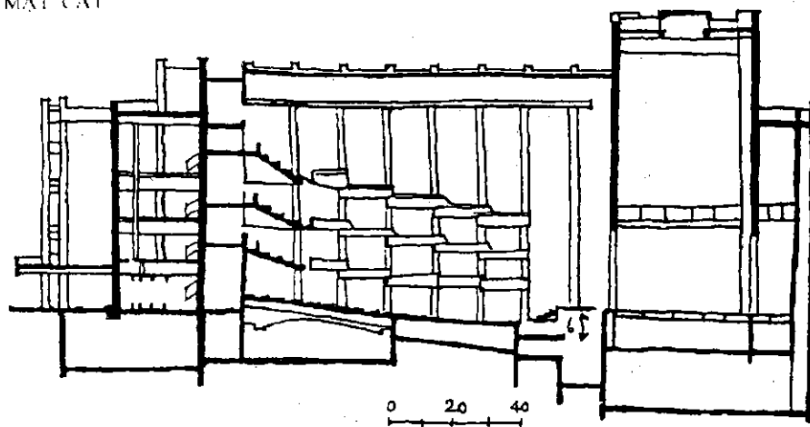
MẶT CẮT
