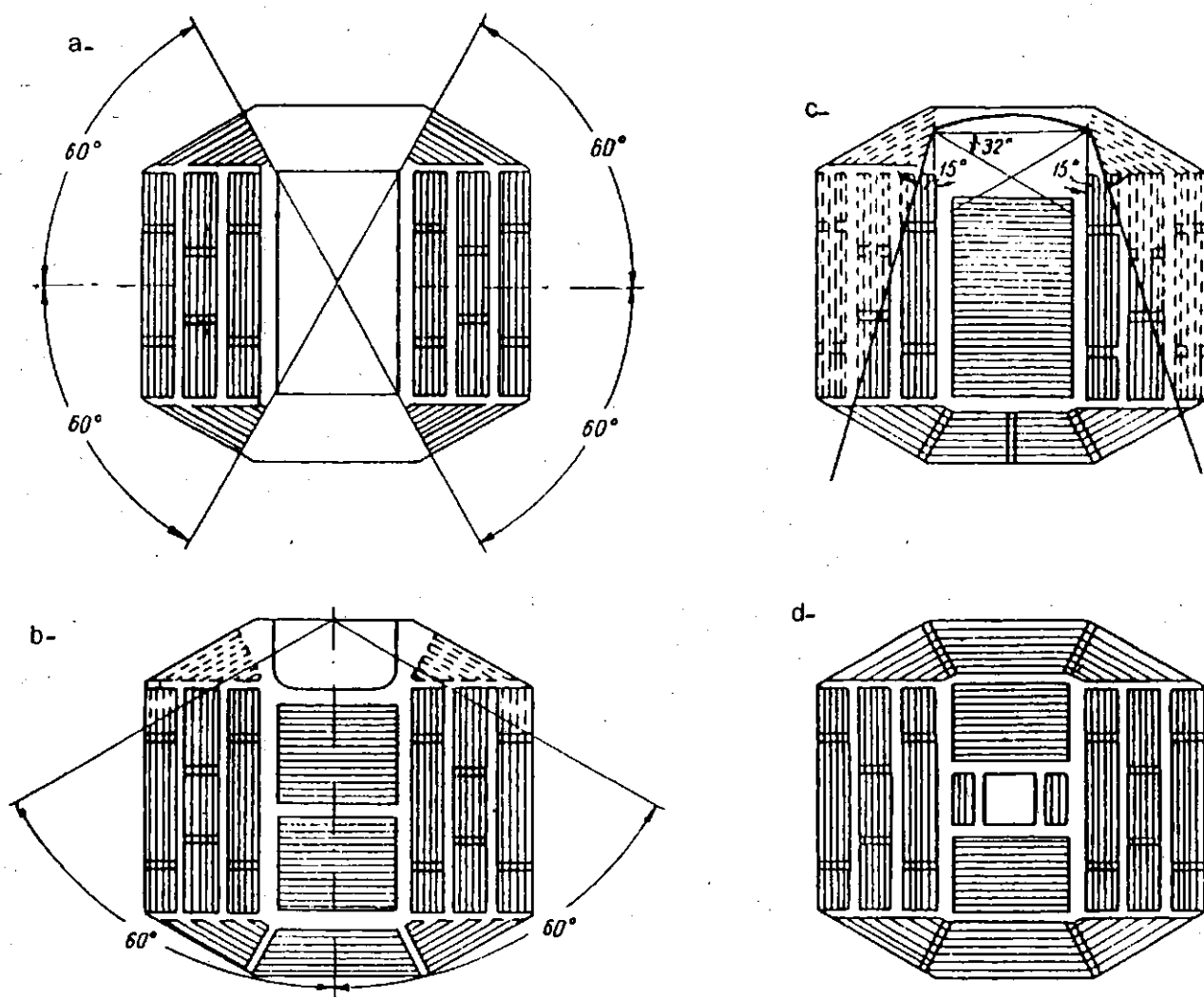
Hình 7.10 : Tham số bố trí chỗ ngồi cho khán giả trong phòng thi đấu thể thao và xem biểu diễn.
