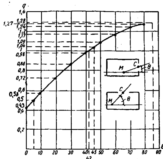
Hình 8.31 : Đồ thị để xác định hệ số q
