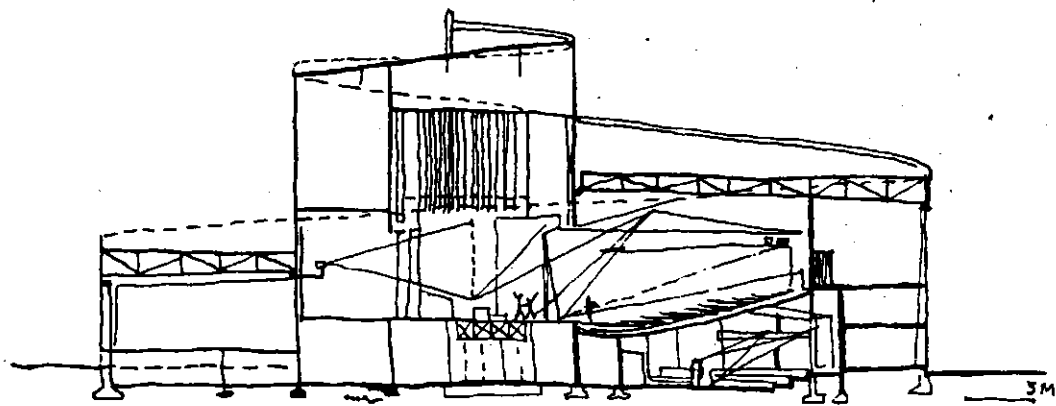
MẶT CẮT
