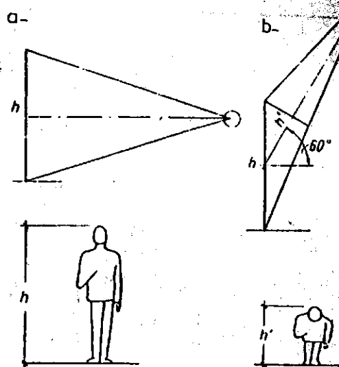
Hình 7.2 : Tỷ lệ của đối tượng quan sát tùy thuộc vào góc nhìn theo phương thẳng đứng
