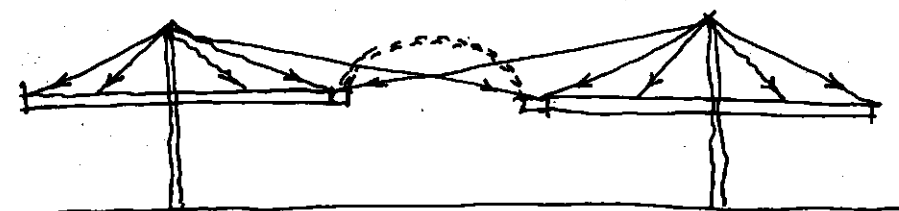
Hình 6.21 : Dây treo miếng cứng
