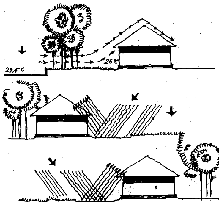
Hình 2.12 : Cây xanh - bãi cỏ giảm nhiệt do bức xạ mặt trời
