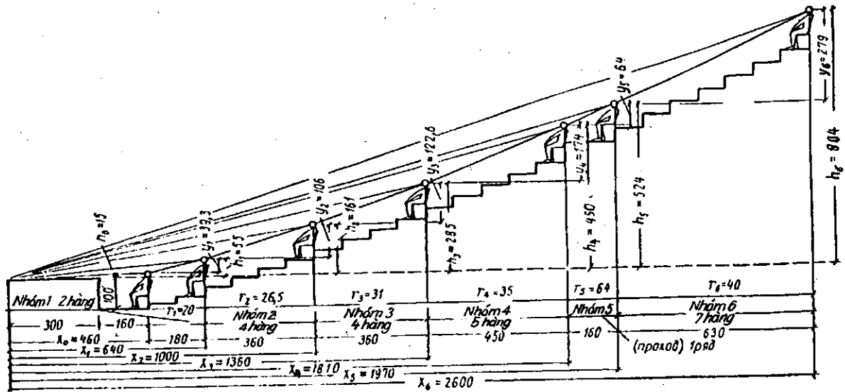
Hình 7.20 : Vẽ mặt cắt nâng cao các hàng ghế theo đường gãy khúc.
