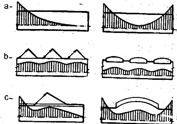
Hình 8.28 : Các đường cong chiếu sáng tự nhiên trong phòng a. Cửa bên ; b. Cửa mái ; c. Hồn hợp cả cửa bên và cửa mái.
