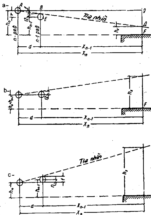
Hình 7.22 : Các sơ đồ kiểm tra điều kiện nhìn rõ
