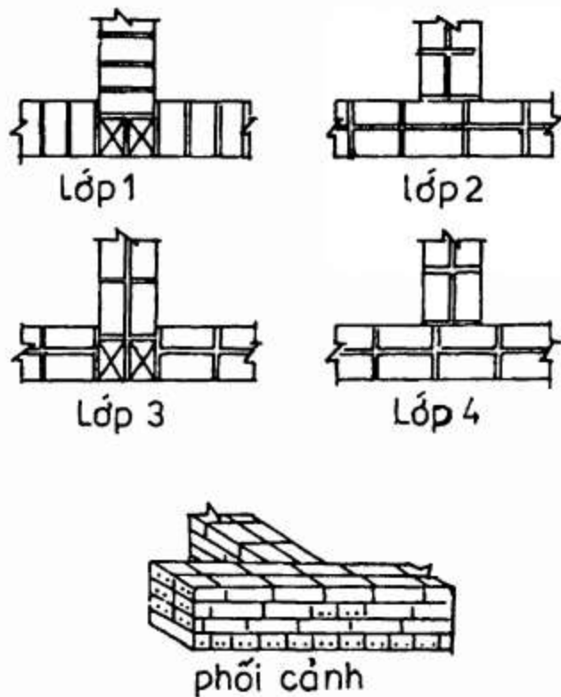
Hình 4.3: Cấu tạo tường chữ đinh 220 (T)
