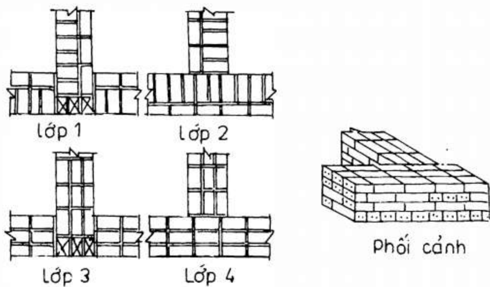
Hình 4.6: Cấu tạo tường chữ đinh 330 (T)
