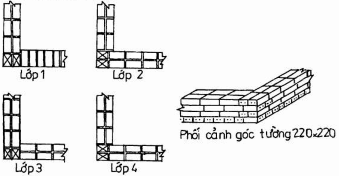
Hình 4.2: Cấu tạo góc tường 220
