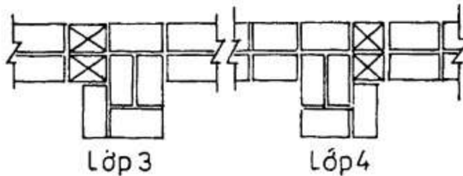
Hình 4.8: Cấu tạo trụ liền tường (trụ 220×220 tường 110; trụ 330×330 tường 220; trụ 330×450 tường 220)
